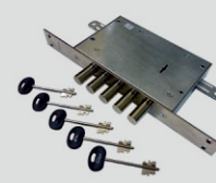
Сувальдный замок Mettem 3B1 341.1.1 (Россия)
